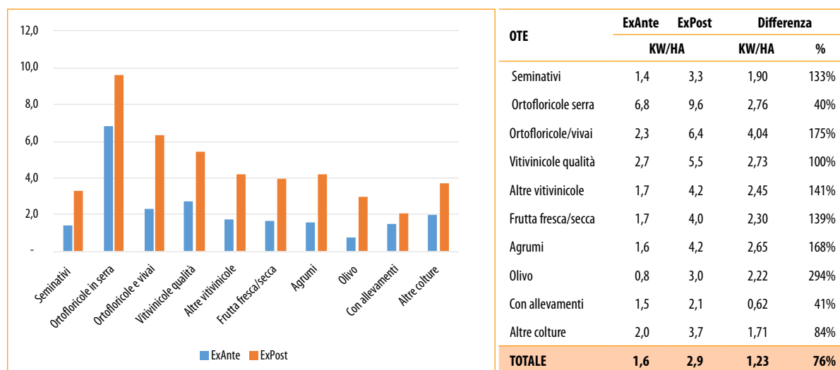
FIG. 44 - POTENZA MACCHINE AZIENDALI PER OTE - FINANZIATE - CONFRONTO EX ANTE/EX POST (KW/HA)
